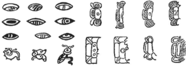
Figura 3. Algunos símbolos Maya representando cero
