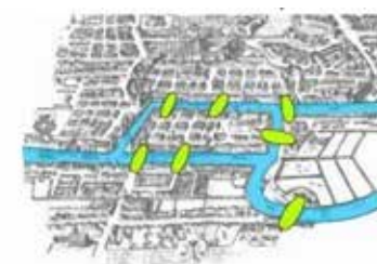
Representación de la ciudad de Königsberg
