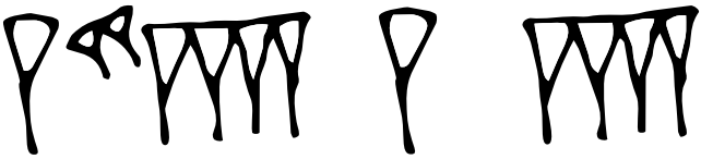
Figura 2. Los números babilónicos 3604 a la izquierda, y 3840 (¿o tal vez 64?) a la derecha
